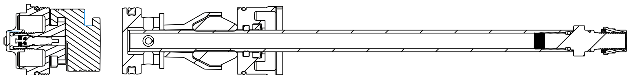
SECTION A-A
