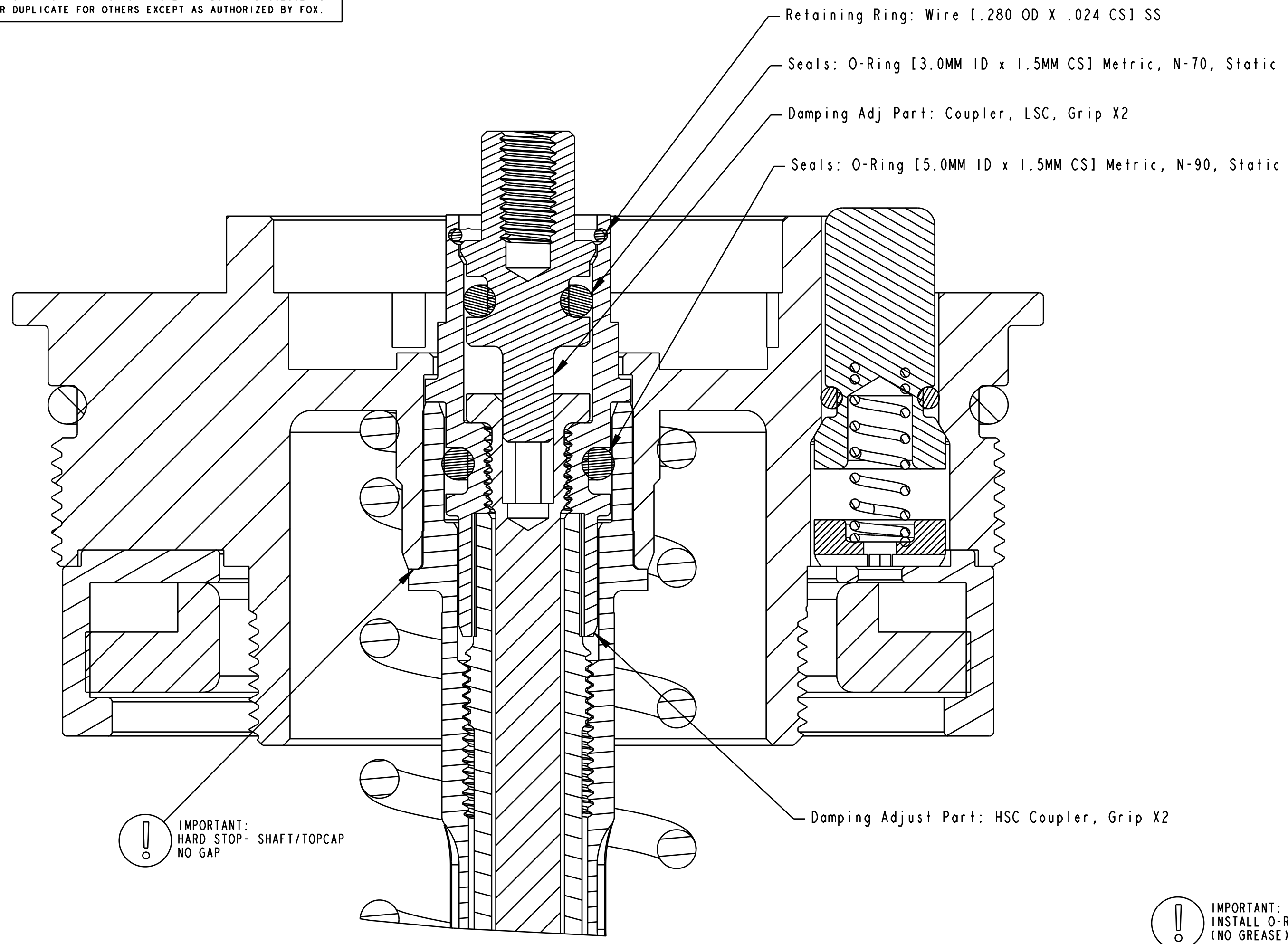
DETAIL Y SCALE 6:1
