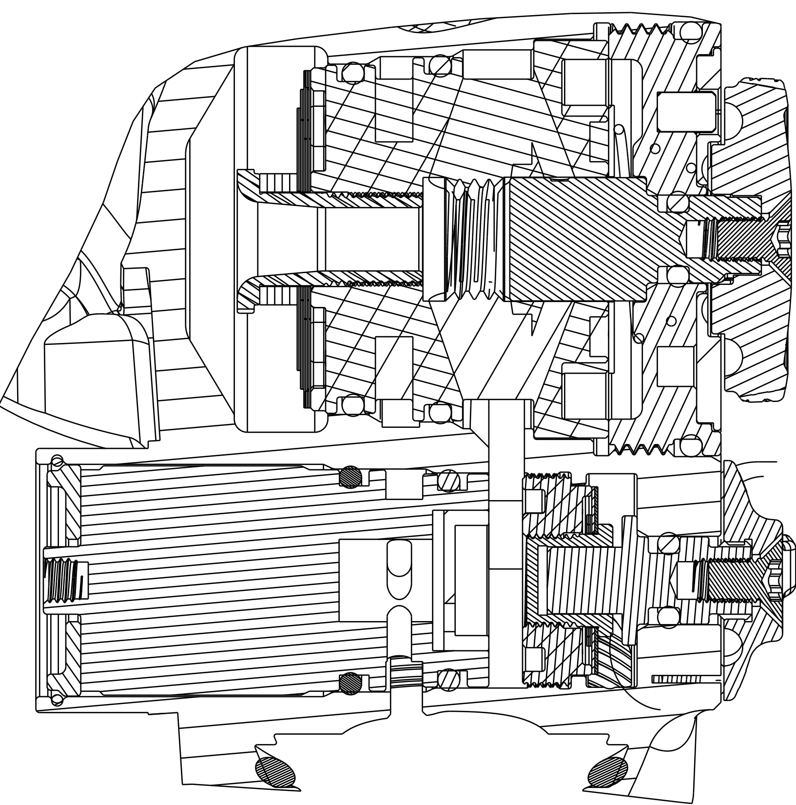
SECTION A-A SCALE 4:1
