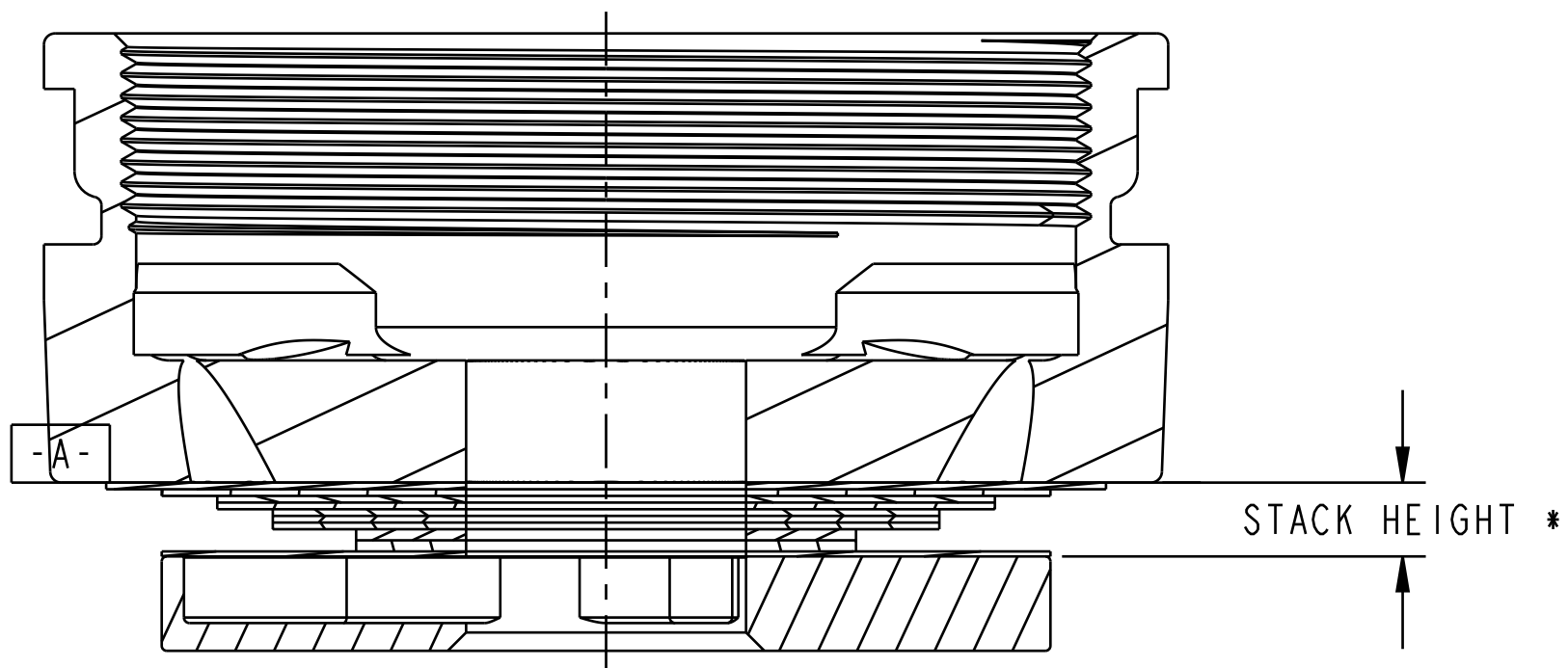
SECTION A-A SCALE 6.000
