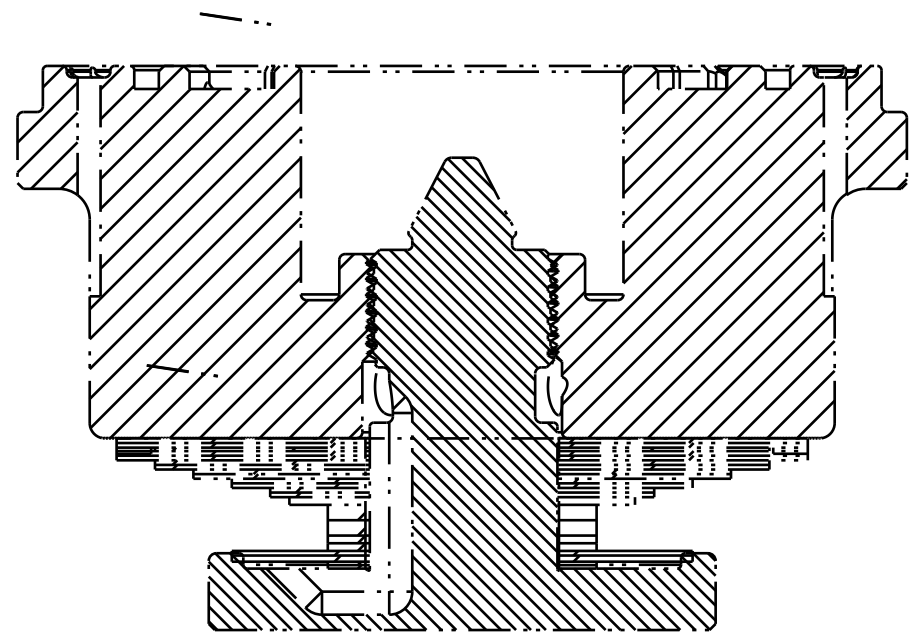
SECTION A-A SCALE 4:1
