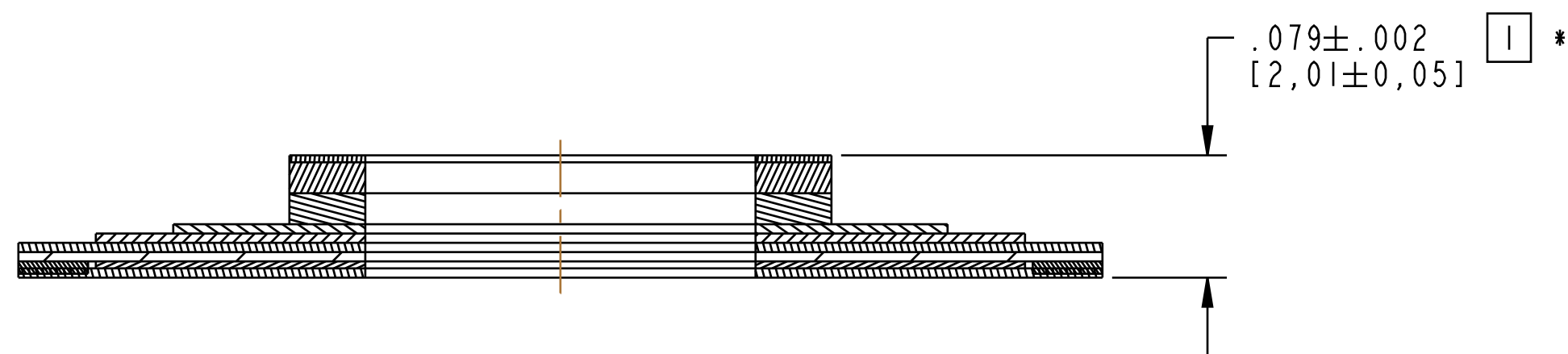
SECTION A-A SCALE 10:1
