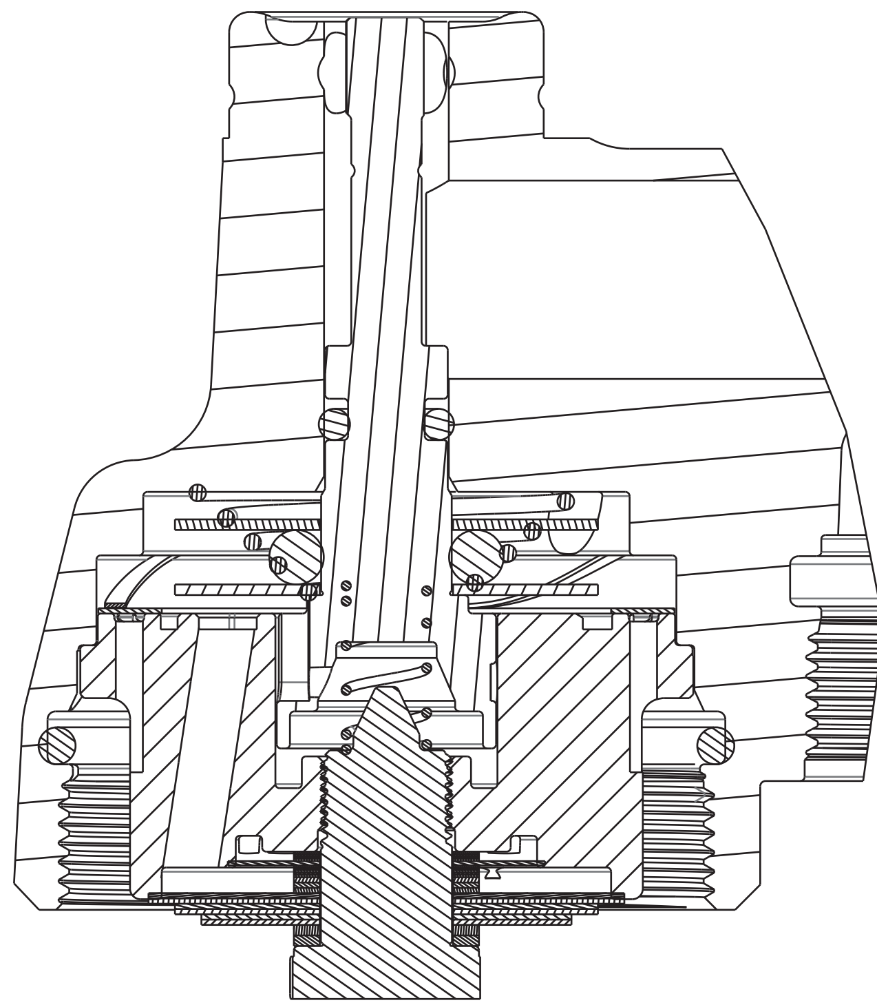
SECTION A-A SCALE 4:1
