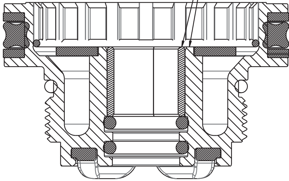
SECTION A-A SCALE 3:1
