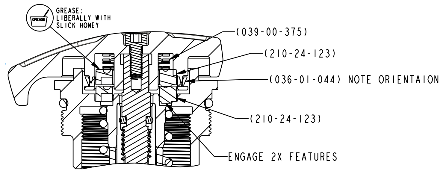
SECTION A-A SCALE 2.500
